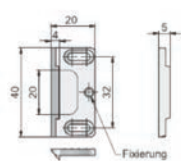
Schließwinkel
