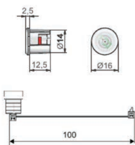
Anzeigeeinheit
