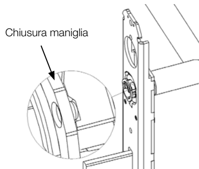
Posizione corretta della chiusura della maniglia quando chiusa
