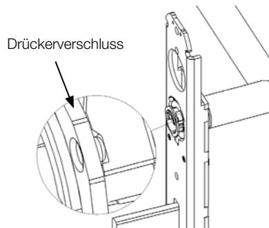
Korrekte Position des Drückerverschlusses im geschlossenen Zustand
