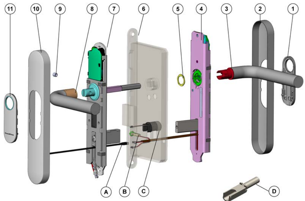
SmartHandle-Komponenten (SnapIn)
